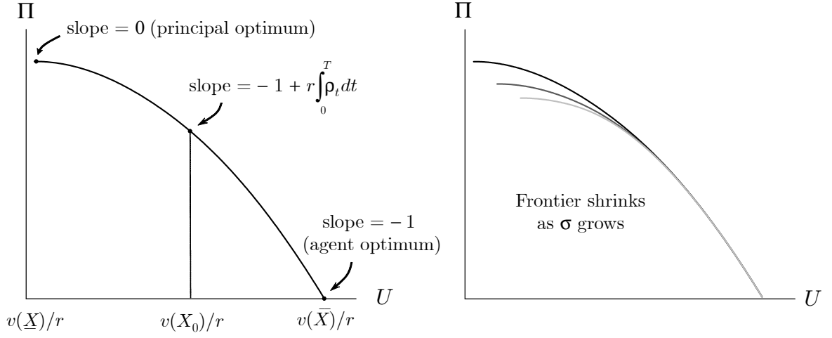
Panel A. Pareto frontier.
